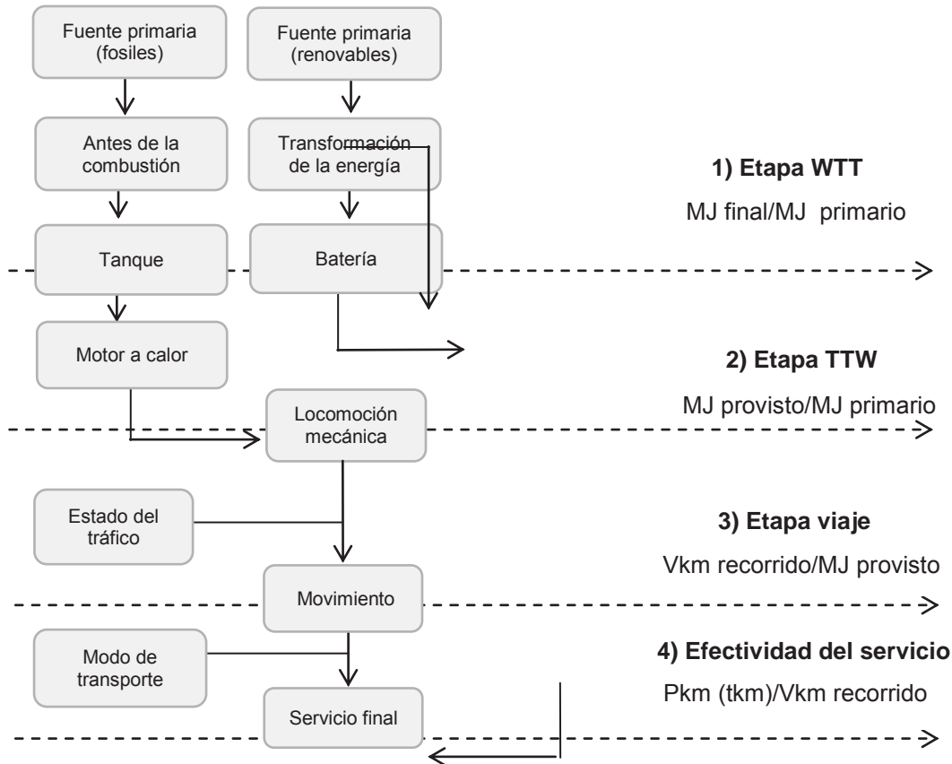
DIAGRAMA 8 ETAPAS BÁSICAS EN EFICIENCIA ENERGÉTICA EN EL TRANSPORTE
