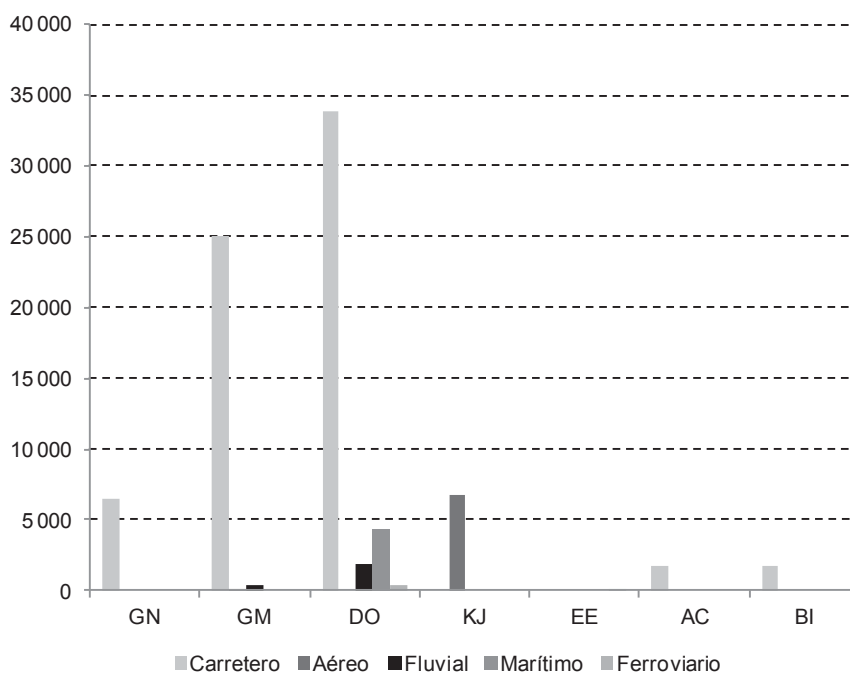
GRÁFICO 35 DEMANDA DE ENERGÍA DEL SECTOR DE TRANSPORTE DE COLOMBIA, 2009
