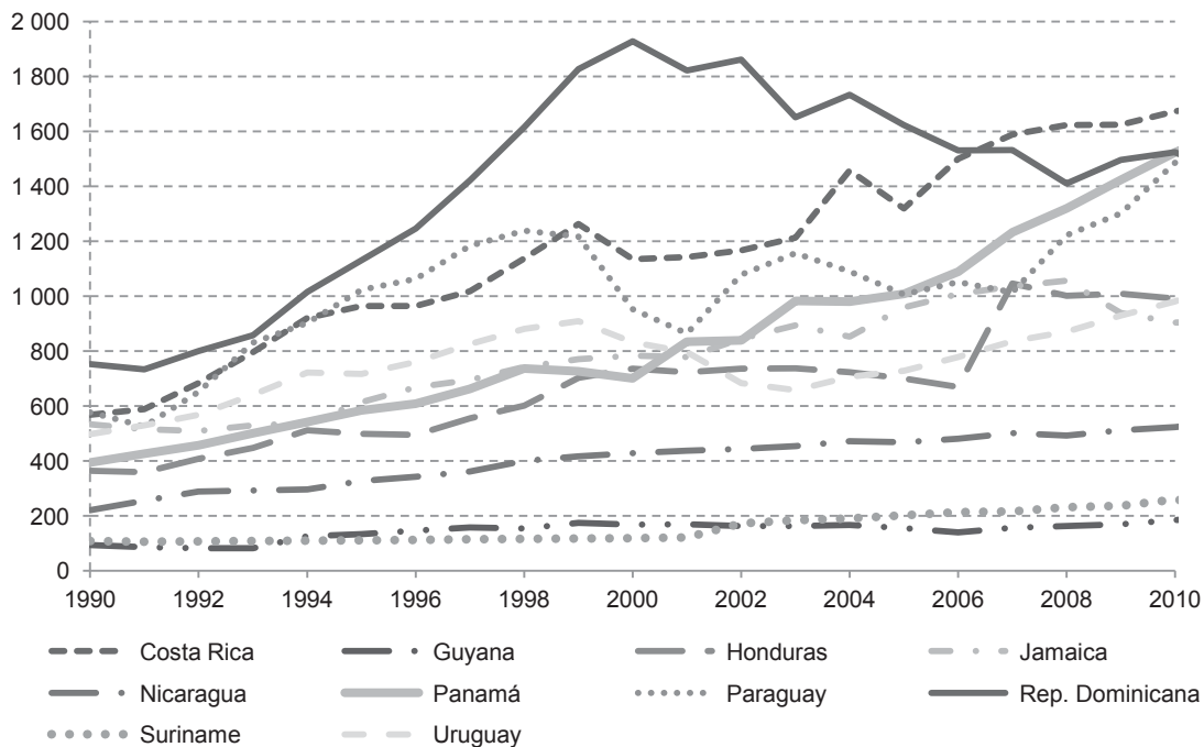
GRÁFICO 24 CONSUMO ENERGÉTICO DEL SECTOR TRANSPORTE, PAÍSES CON MENOR CONSUMO (Países con consumo inferior a 2.000 ktep/año)
